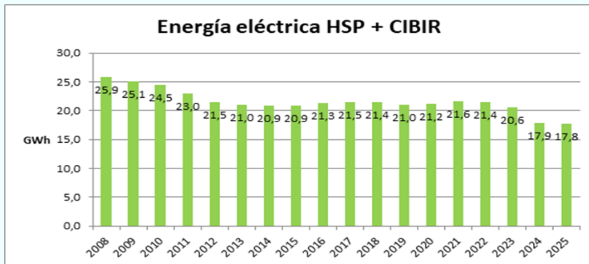
Energía eléctrica (GWh) consumida en Hospital Universitario San Pedro 2008-2025
